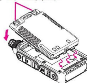
Защелки аккумулятора
